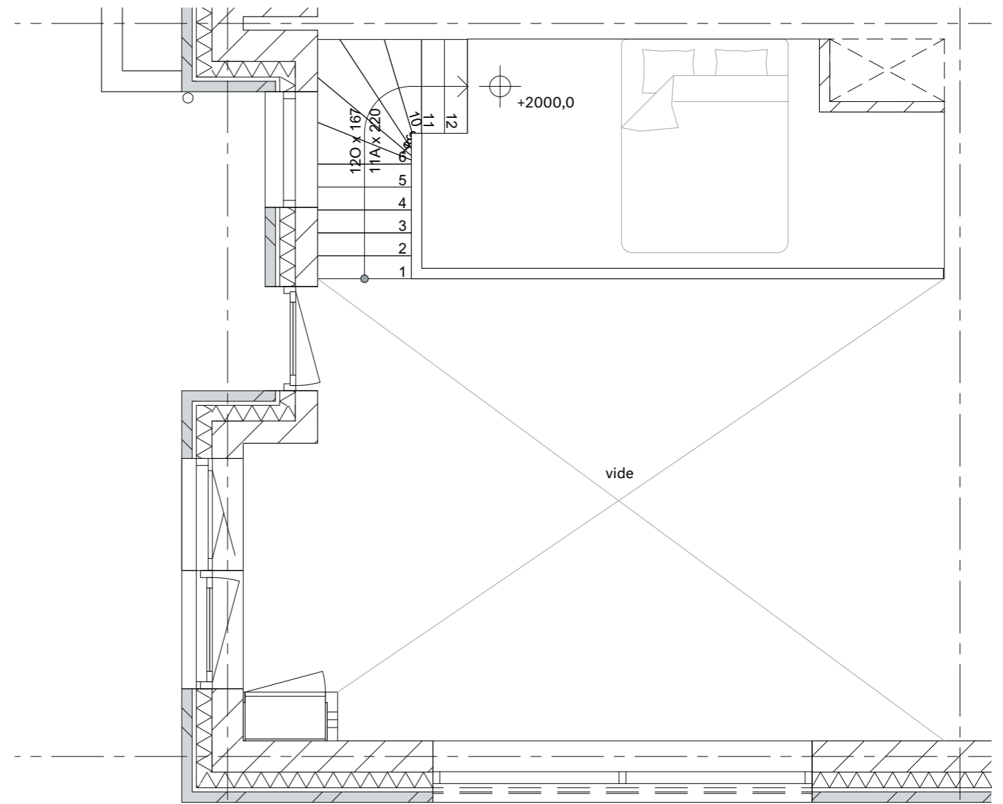
Tussenverdieping
