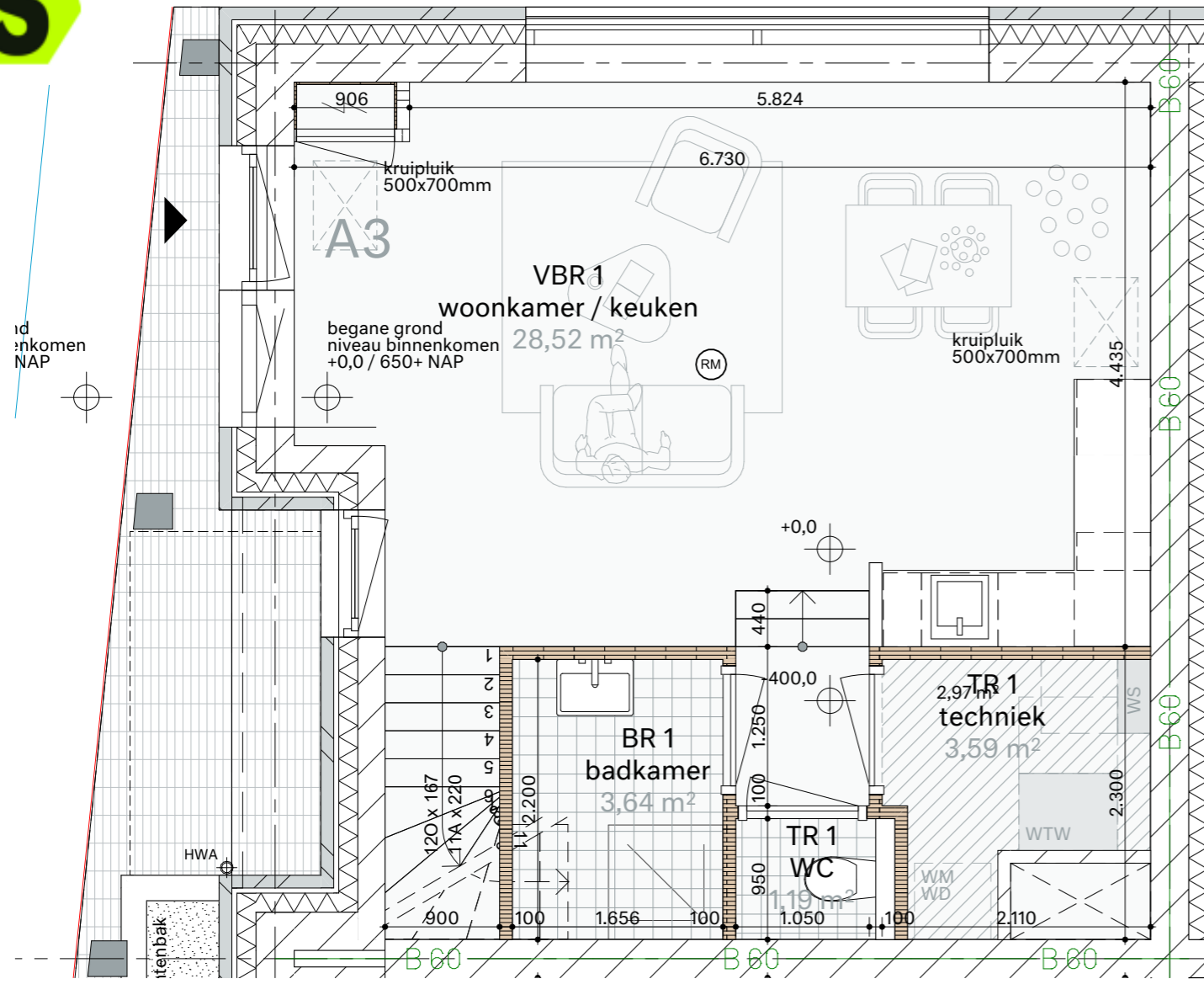
Begane grond
