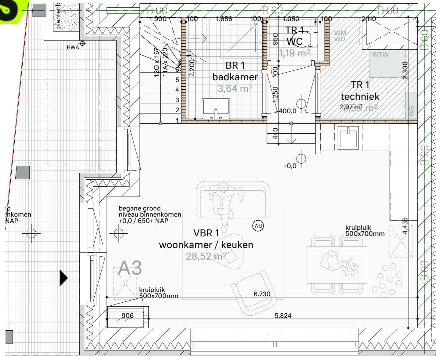
Begane grond
