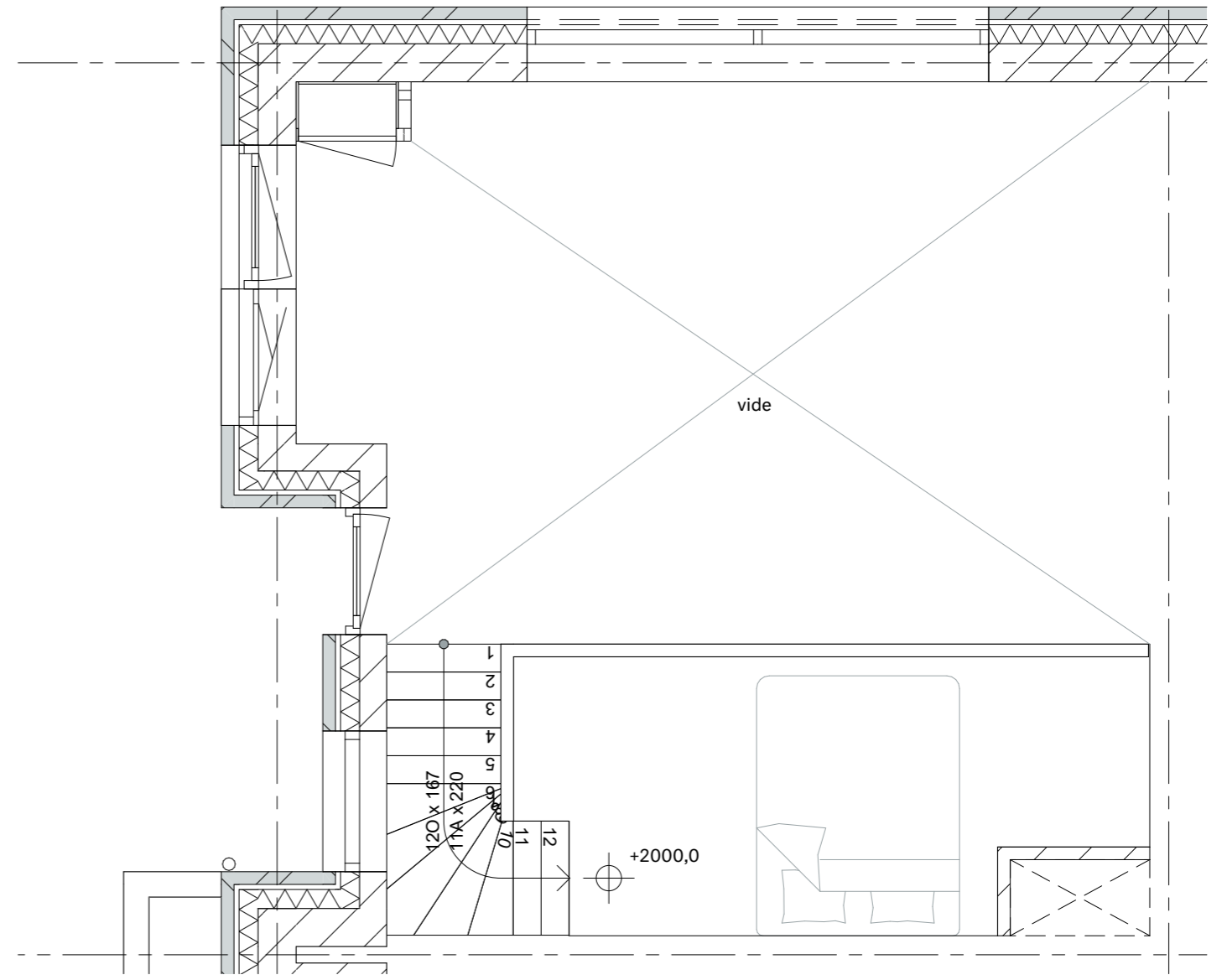
Tussenverdieping
