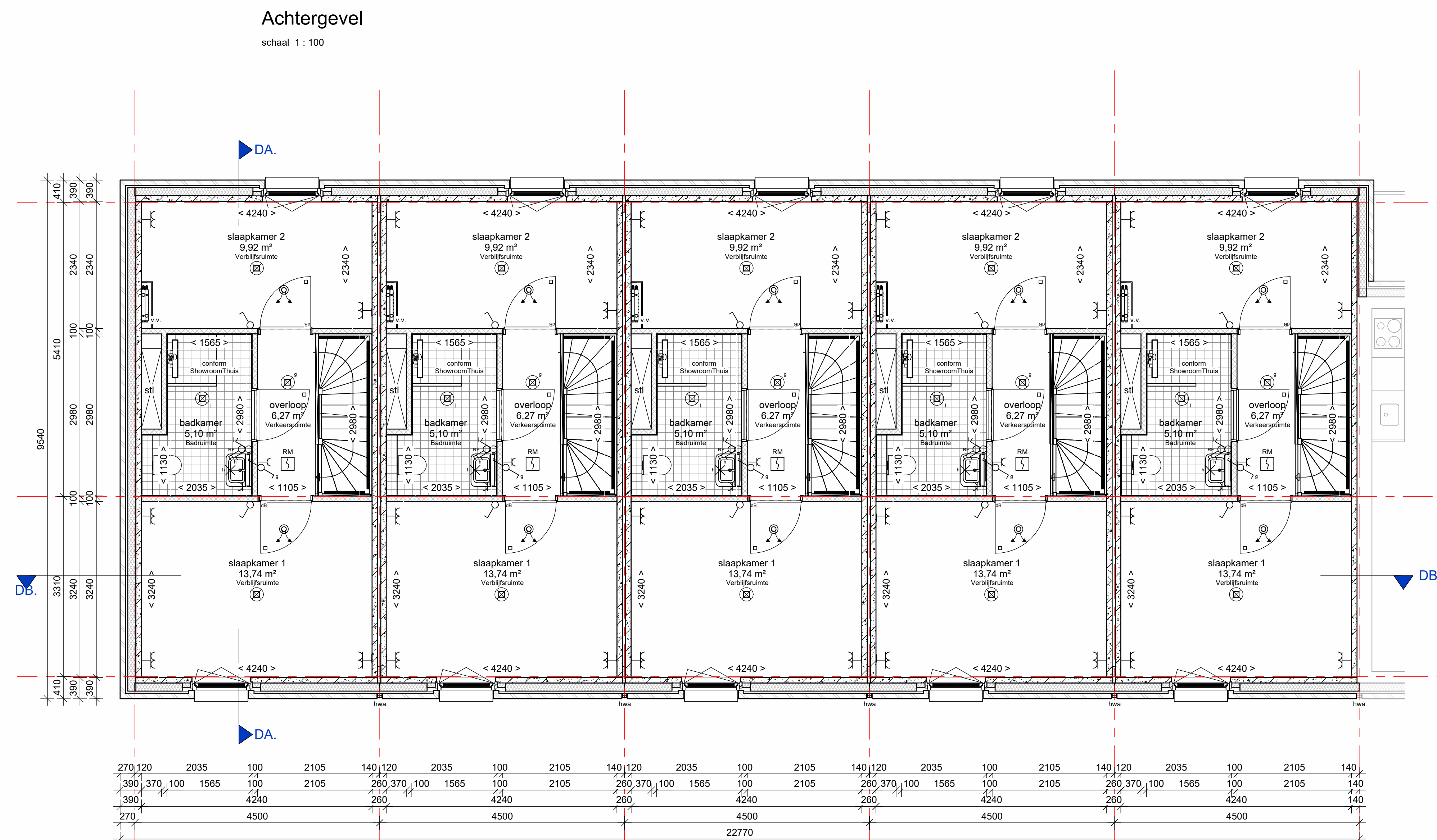
2e verdieping
