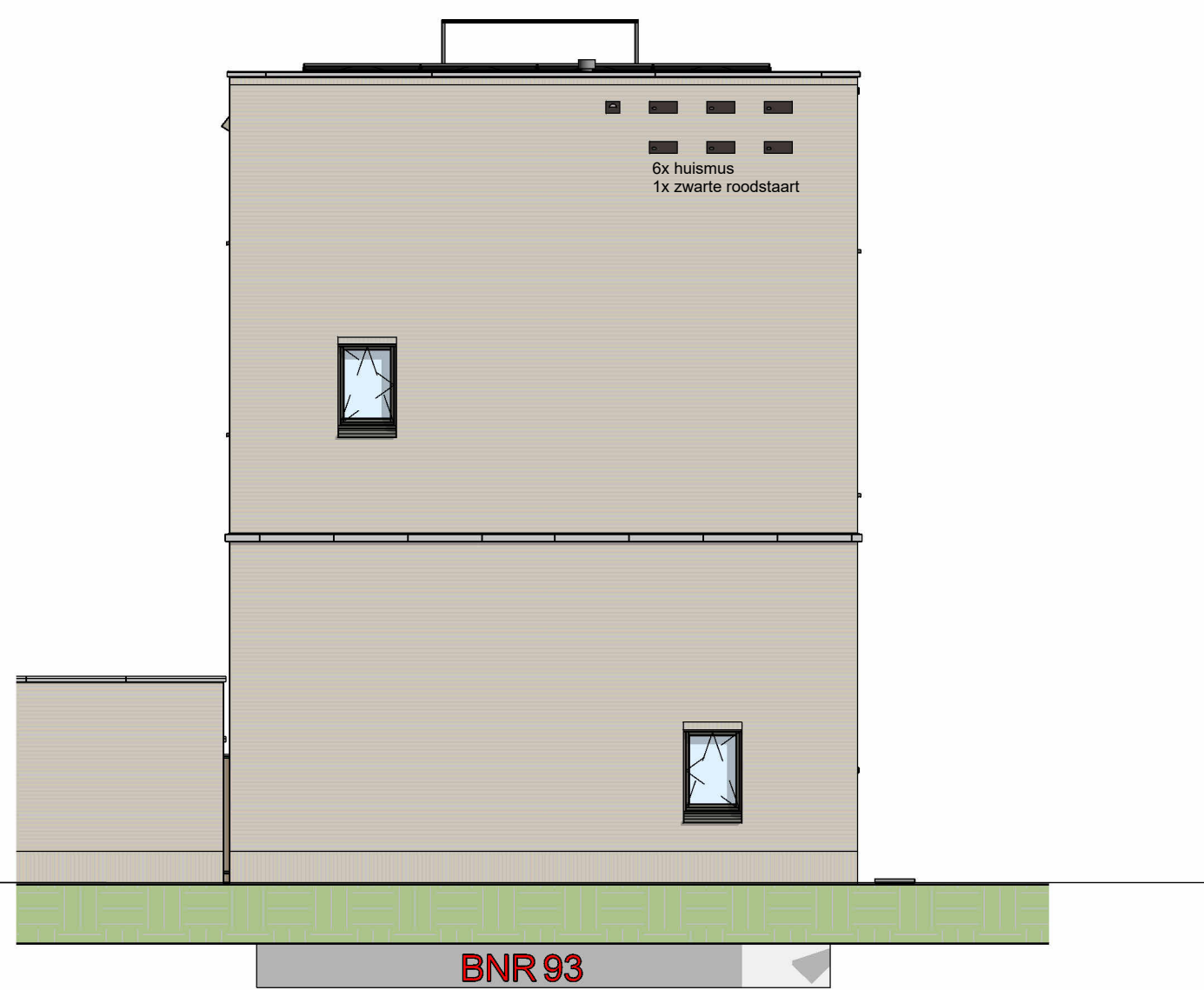
Linker zijgevel
