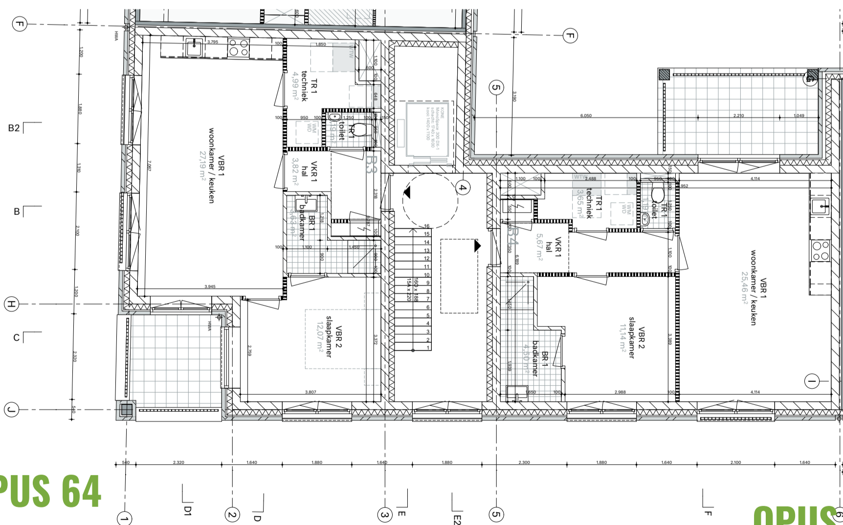
3E VERDIEPING
