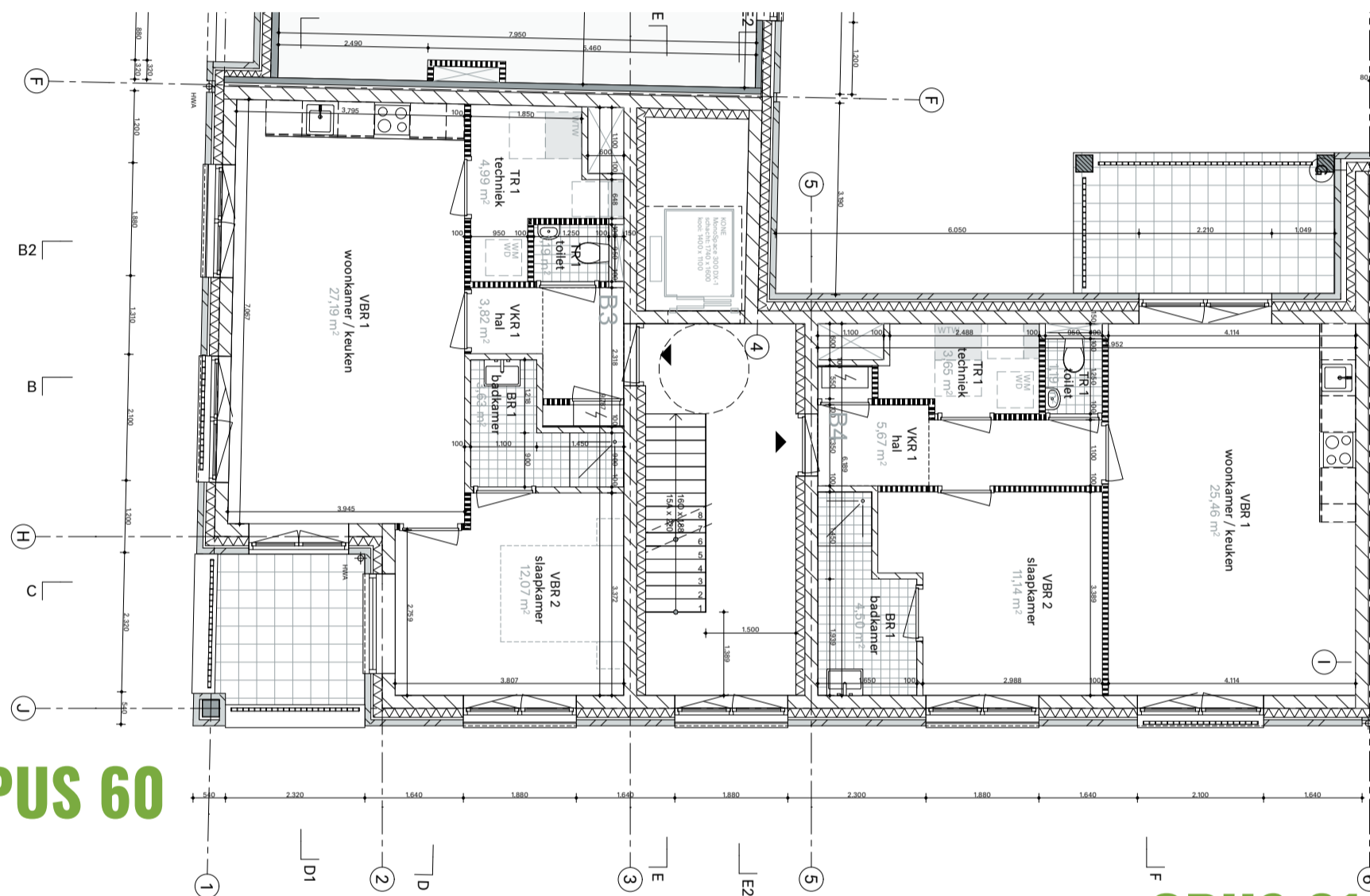
1E VERDIEPING
