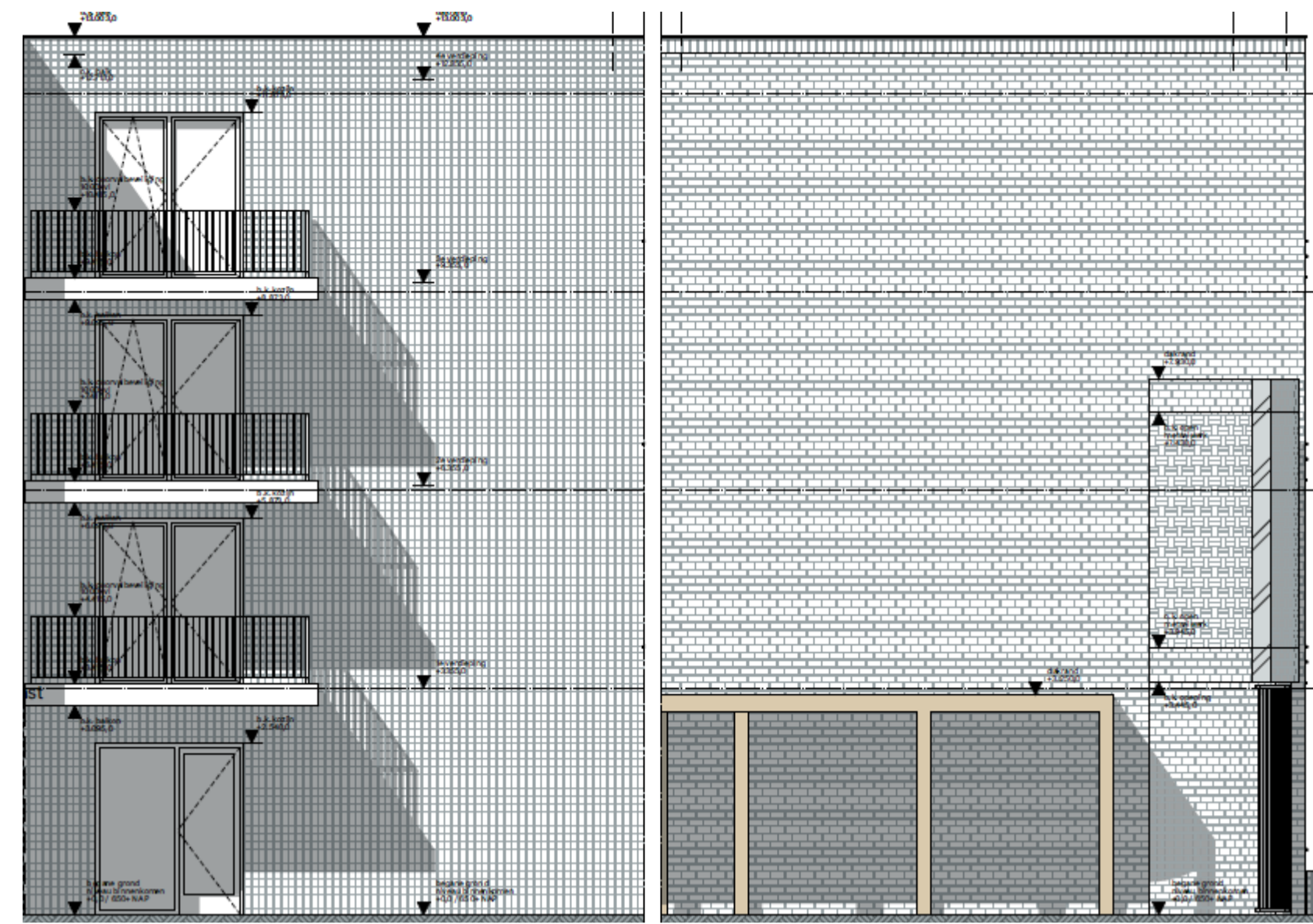
WESTGEVEL
