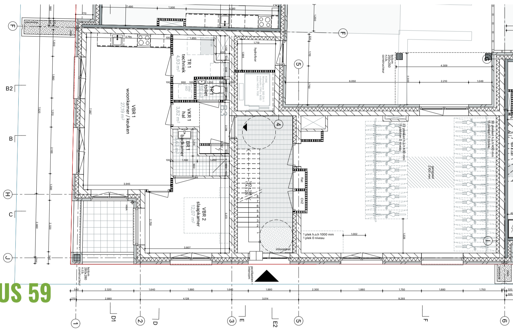
BEGANE GROND
