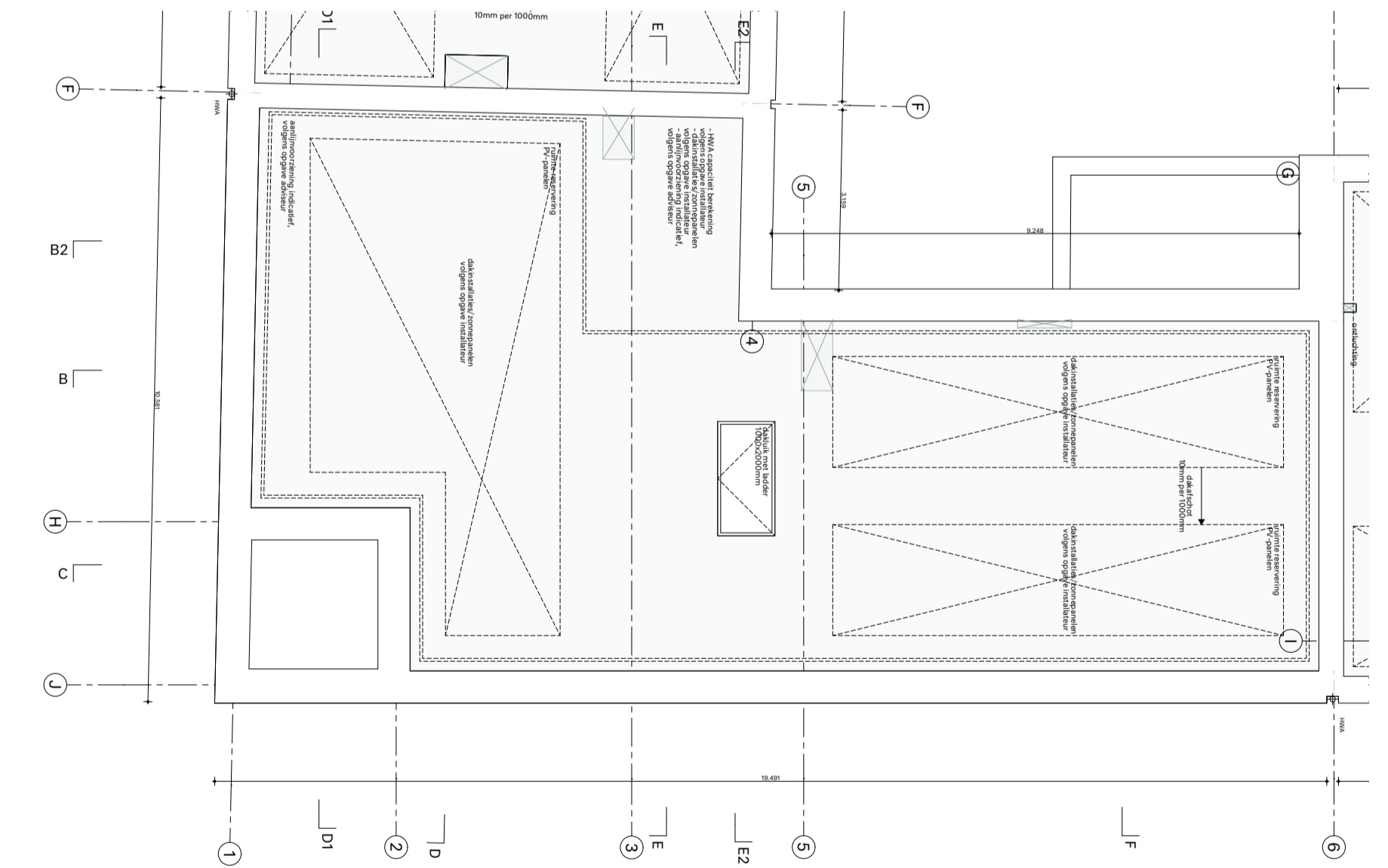
DAKAANZICHT
