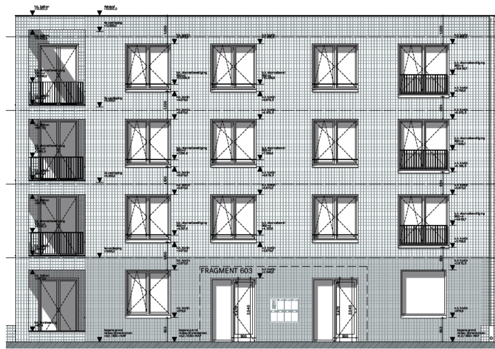
OOSTGEVEL
