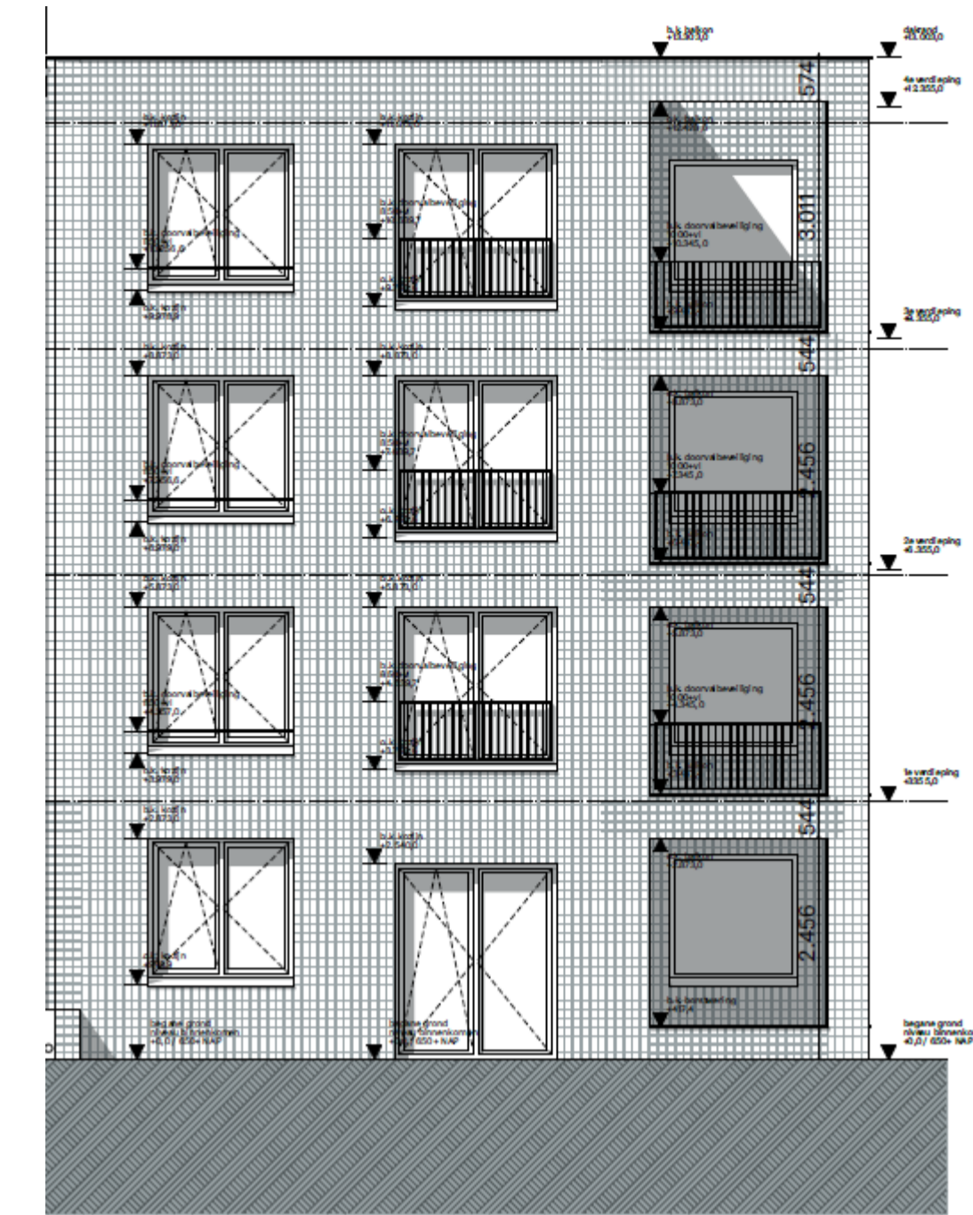
ZUIDGEVEL
