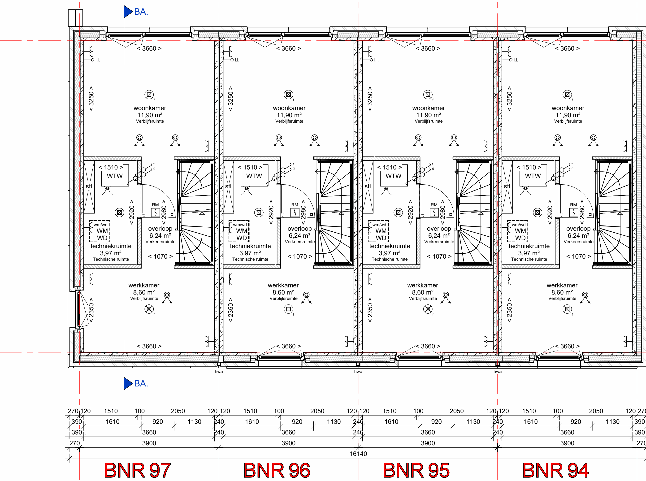
1e verdieping schaal 1 : 50
