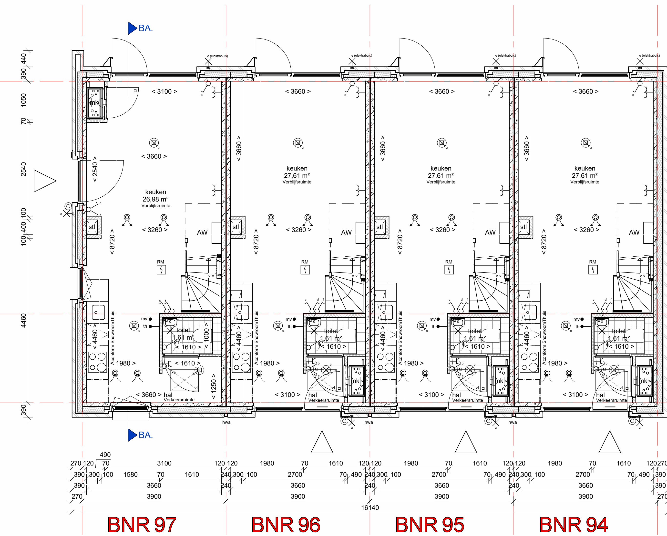
Begane grond schaal 1 : 50
