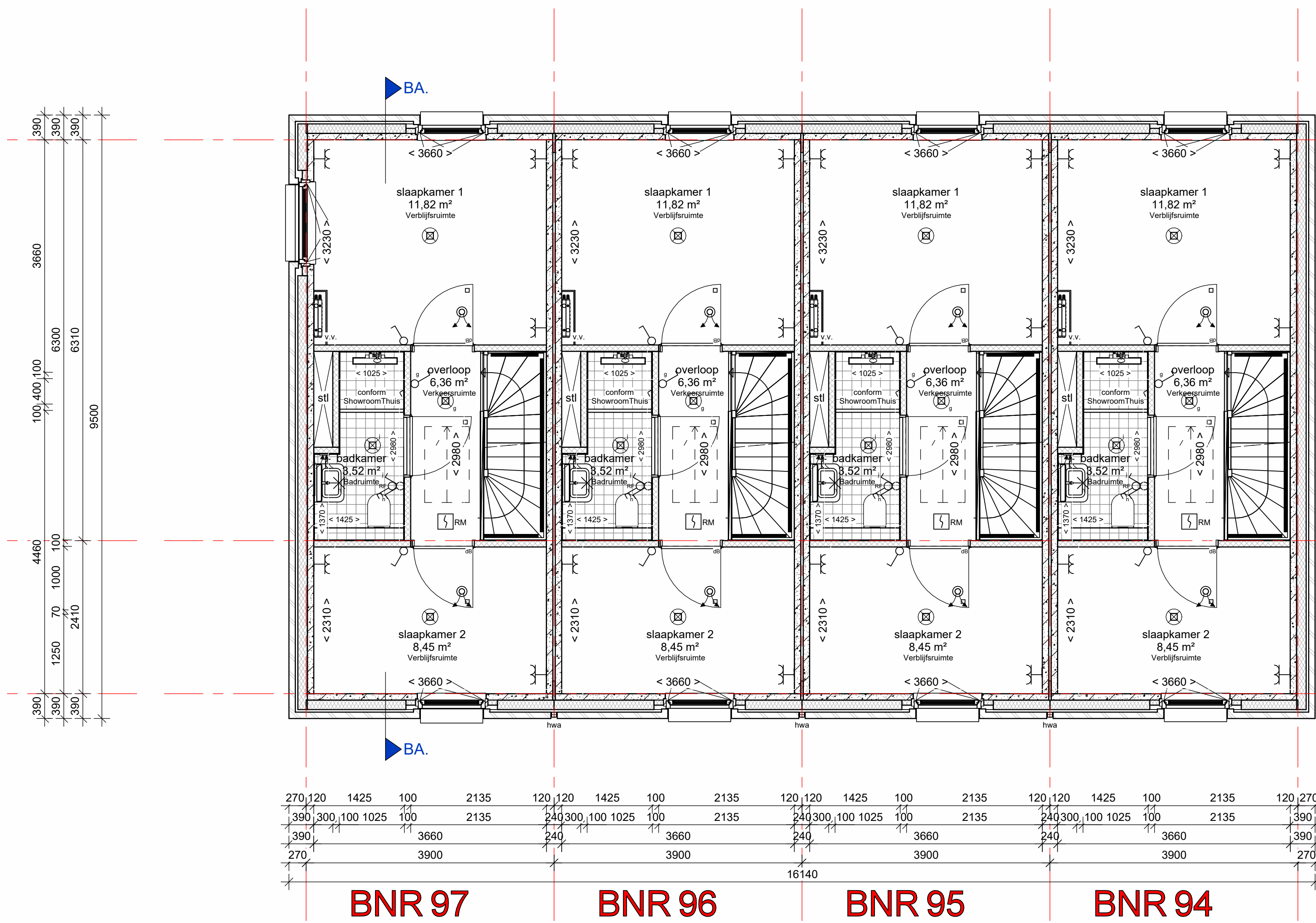
2e verdieping schaal 1 : 50
