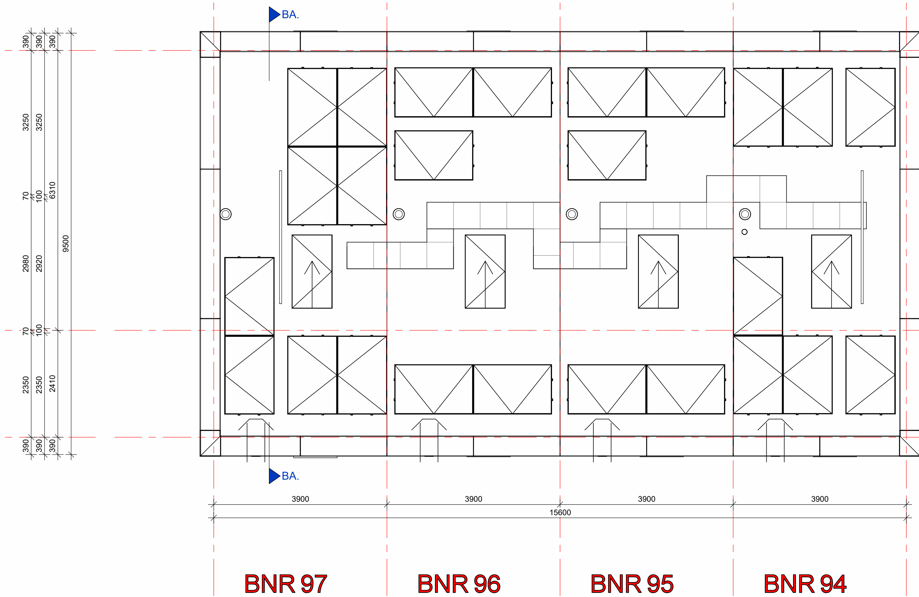
Dakoverzicht schaal 1 : 50
